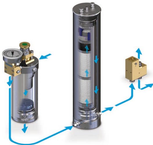
Фильтровальная система P 41
