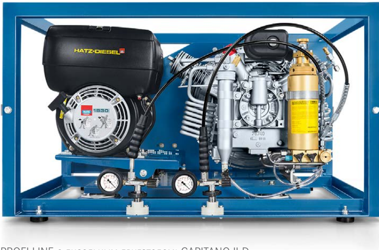
PROFI LINE с дизельным двигателем: CAPITANO II-D
